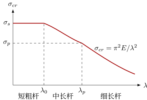
图 18: 临界应力总图
