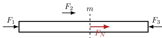
图 2: 轴向杆截面法示意
