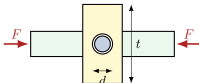
销钉连接：剪切面与挤压投影面需分别识别
