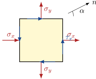
图 14: 平面应力状态与斜截面外法线
