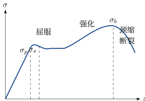
图 3: 低碳钢拉伸应力-应变曲线示意
