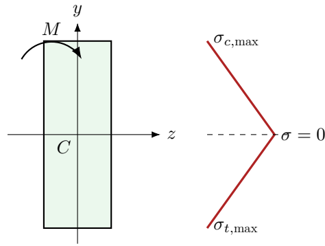
线性正应力分布
